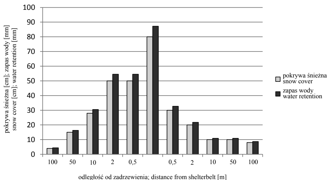
Rys. 1. Akumulacja śniegu i wody w zadrzewieniu „Wysokość” (grudzień 1998) Fig. 1. Snow and water accumulation in shelterbelt “Wysokość” (December 1998).
