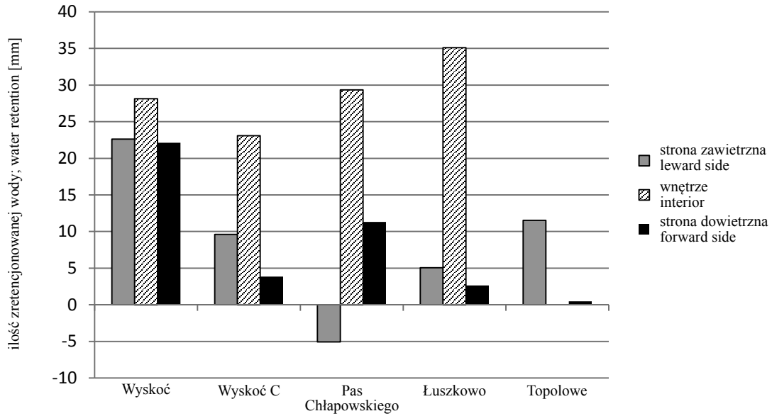
Rys. 3. Wysokość słupa wody (mm) zatrzymanej przez badane zadrzewienia w wyniku akumulacji pokrywy śnieżnej Fig. 3. High of water layer (mm) accumulated in snow cover by studied shelterbelts.
